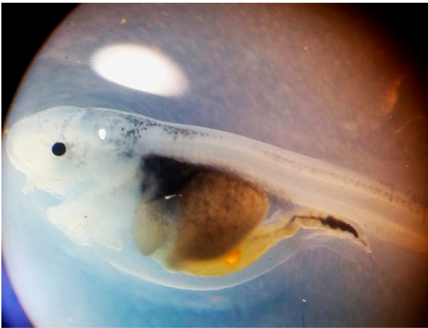
Рис. 2. Предличинка веслоноса
