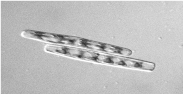
Рис. 1. Climaconeis scalaris (BRÉBISSEON) E.J. COX
