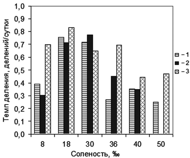
Рис. 2. Темп деления клеток Climaconeis scalaris (BRÉBISSE) E.J. COX:
