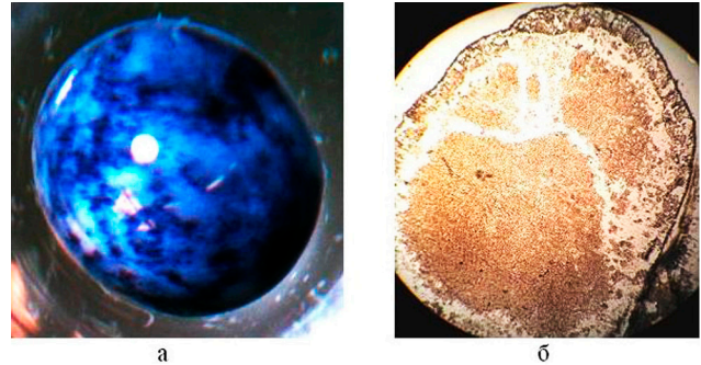
Рис. 3. Начало резорбции: а) мраморная окраска ооцита, июнь, бассейны КЗпО, увеличение 2 × ; б) гистологический препарат, увеличение 20 ×
