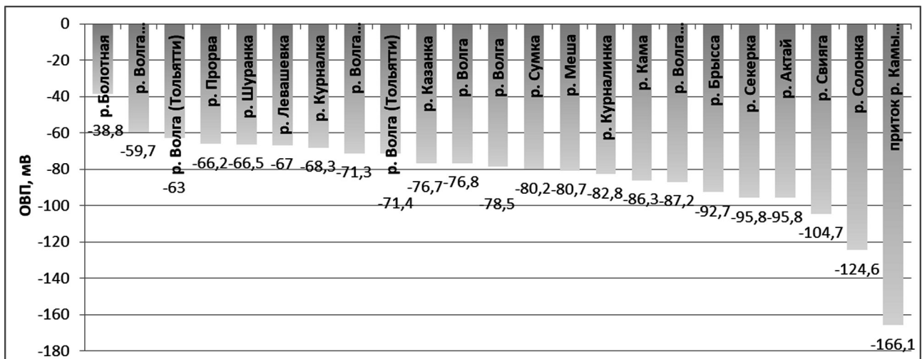
Рис. 2. Изменения ОВП в реках Республики Татарстан
